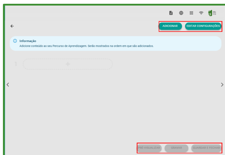
Figura 67: Editor de Percurso de Aprendizagem
