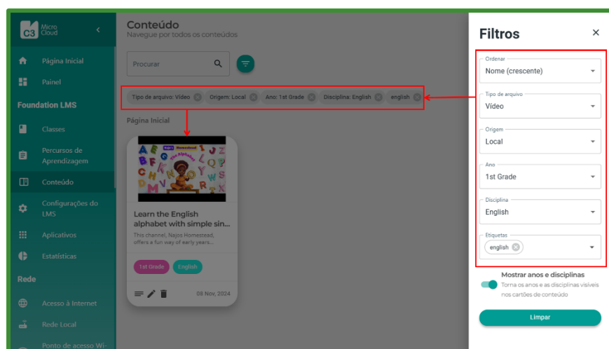
Figura 31: Filtro Aplicado
