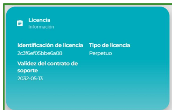
Figura 7: Painel - Licença
