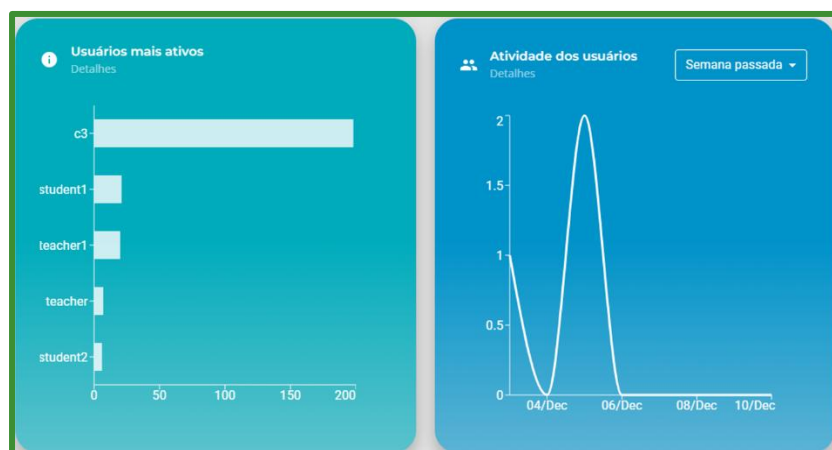
Figura 109: Estatísticas – Utilizadores
