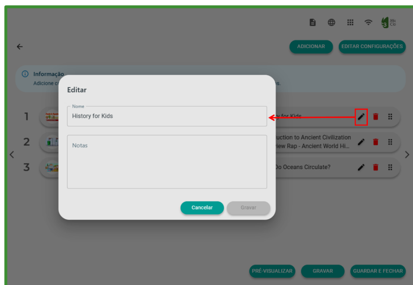
Figura 94: Editar Conteúdo
