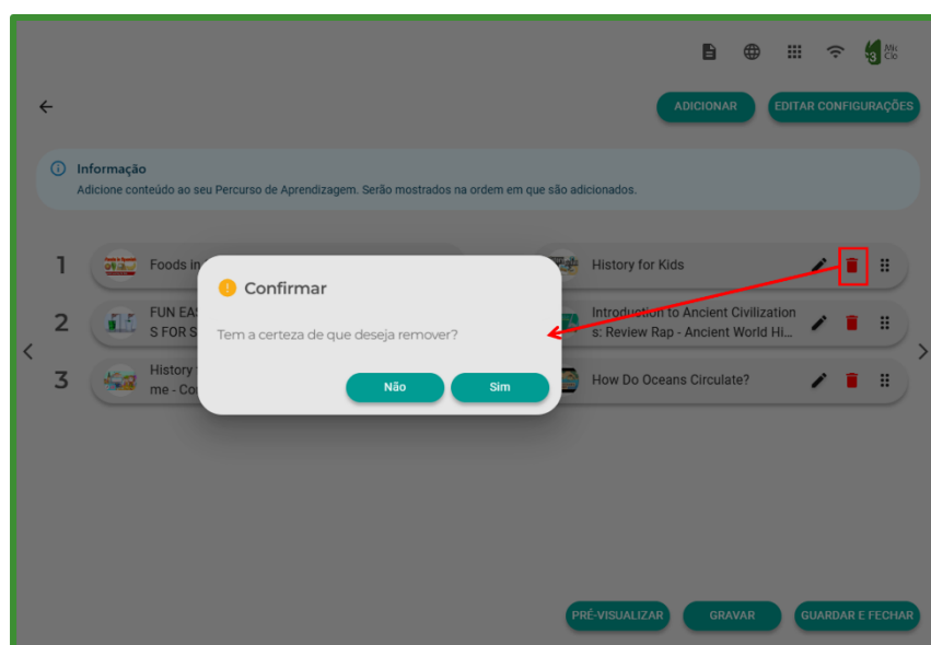
Figura 95: Aviso de Eliminação de Conteúdo
